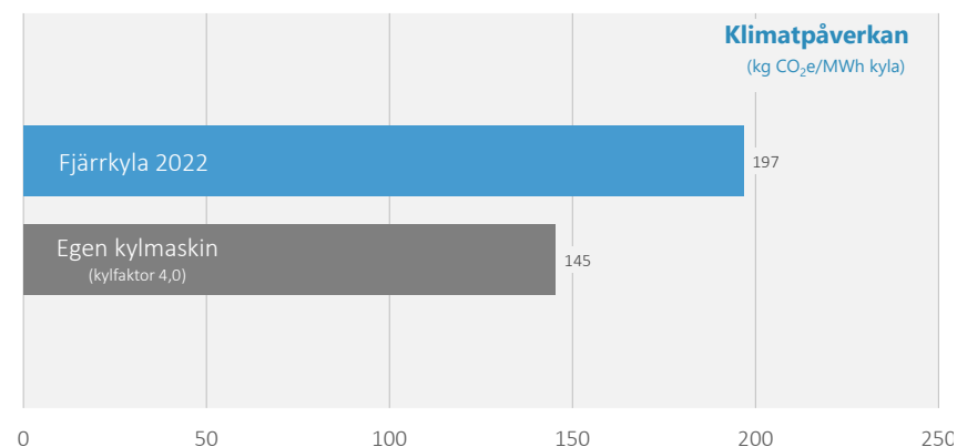
Figur 9 En fjärrkylakunds klimatpåverkan under 2022 i Kalmar i jämförelse med en ny egen kylmaskin.
