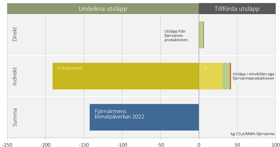
Figur 6 En fjärrvärmekunds klimatpåverkan under 2022 i Kalmar Energis fjärrvärmesystem. Den nedre blå stapeln "Fjärrvärmens klimatpåverkan 2022" är summan av tillförda utsläpp och undvikna utsläpp. Resultatet visar klimatpåverkan från att producera och leverera fjärrvärme fram till kund .
