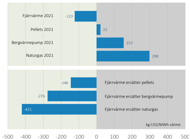
Figur 7 Klimatpåverkan för olika uppvärmningsalternativ 2022. I den övre delen av diagrammet jämförs en fjärrvärmekunds klimatpåverkan i Kalmar Energis fjärrvärmesystem med tre andra tekniker. I den nedre delen av diagrammet visas den resulterande klimatpåverkan då fjärrvärme ersatte någon av de andra uppvärmningsalternativen under 2022.
