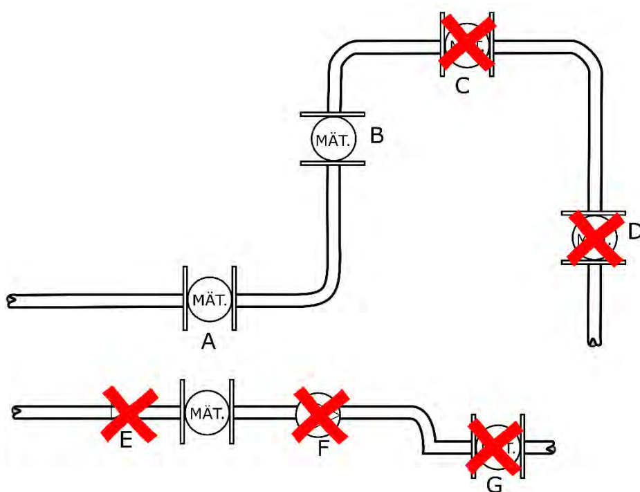
Figur 21. Lämplig placering av flödesgivare
